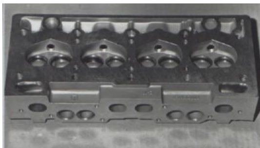
Chiulasa serie Dacia/Renault cu supape paralele (camera de ardere tip "pana") Porturi rotunde Porturi patrute
